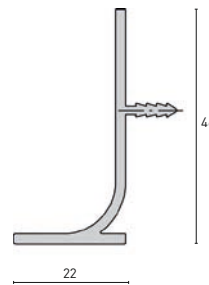
Griffmulde L-Profil vertikal
