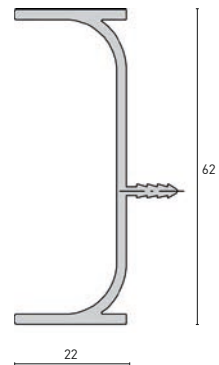
Griffmulde C-Profil vertikal
