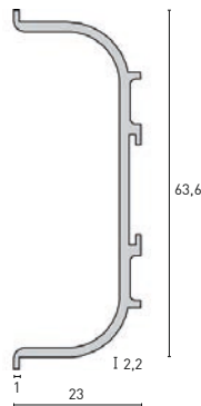
Griffmulde C-Profil horizontal
