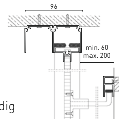
Führungsprofil für hintere Führung
