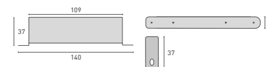
Rollenkästen für die untere Laufrolle
