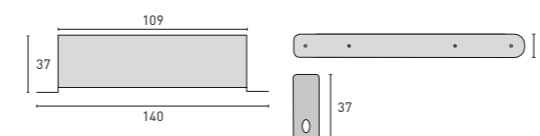
Rollenkasten für die untere Laufrolle
