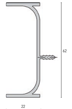
Griffmulde C-Profil vertikal
