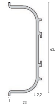
Griffmulde C-Profil horizontal
