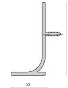
Griffmulde L-Profil vertikal
